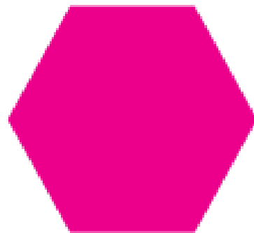
Segi enam
