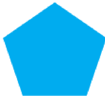
Segi lima
