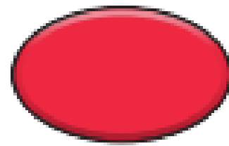
Bentuk lengkung
