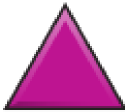
Segitiga
